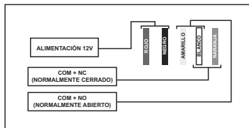
DIAGRAMA DE CABLEADO
